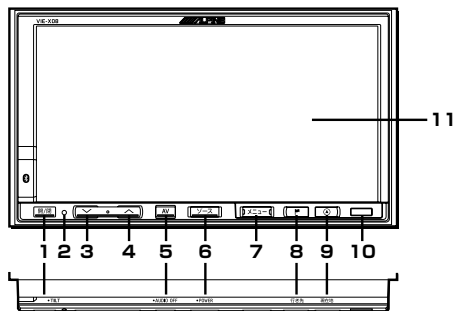
＜本機正面＞
