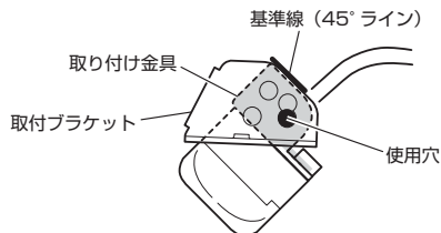
<角度調整と使用穴位置>
