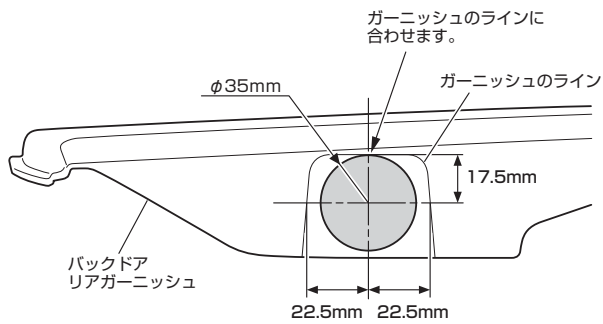
<バックドアリアガーニッシュを表側から見た図>
