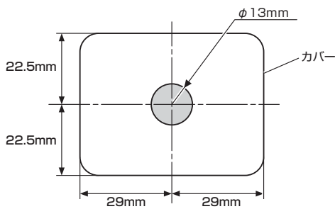
<カバーを表側から見た図>
