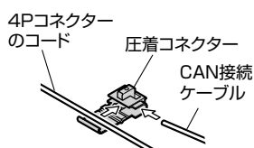
CAN接続ケーブル:緑 4Pコネクタのコード:2番
